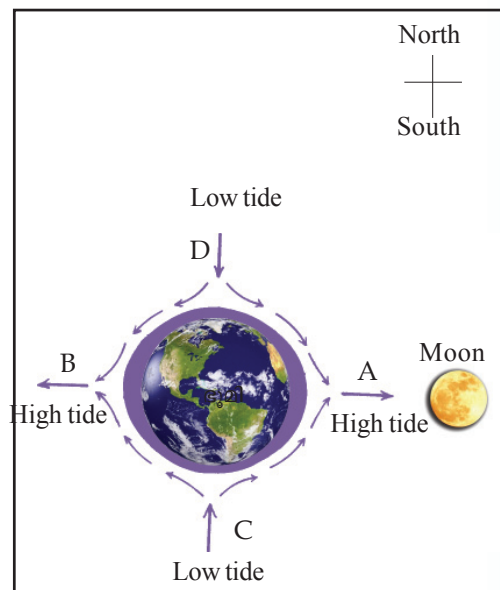
Fig 5.4 Tides
